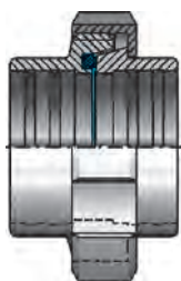
Expanding union 2009 DIN 11851
