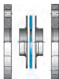
Alu-Losflansch PN 10 DIN EN 1092-1 mit Vorschweißbördel (Vorschweißbördel Edelstahl)
