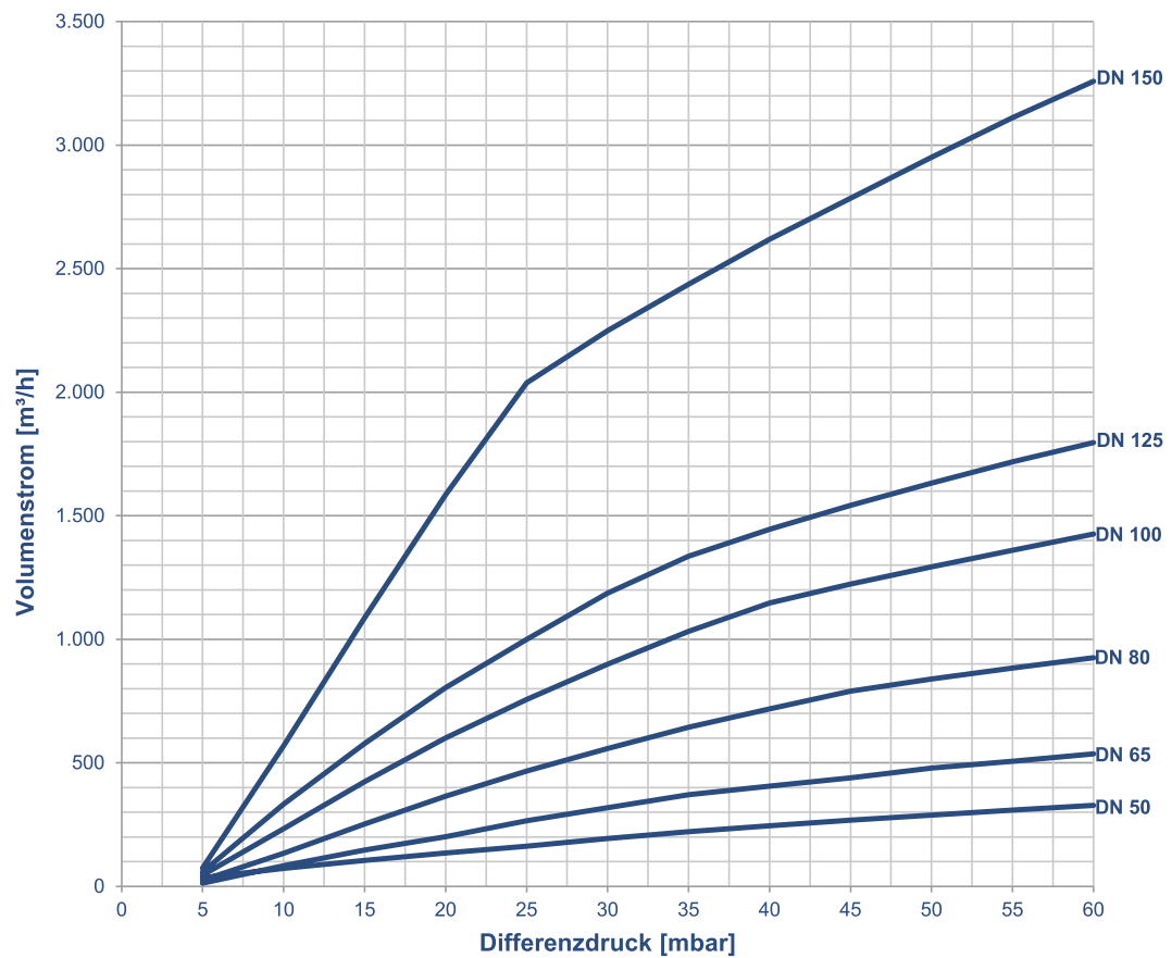
Auslegungsdiagramm Vakuumventil 6160
