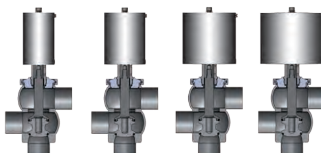
Vier verschiedene Antriebsgrößen für unterschiedliche Anwendungen (Betriebsdruck)
