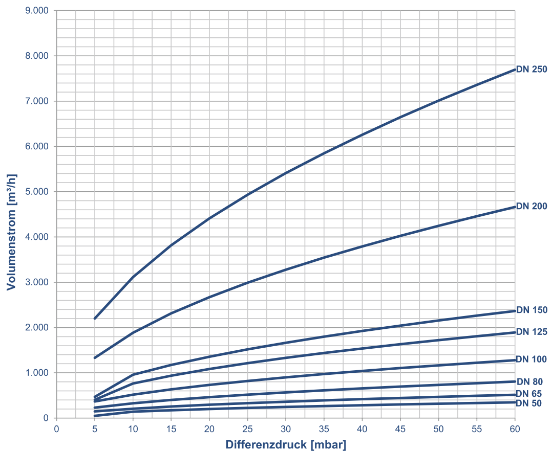
Auslegungsdiagramm Vakuumventil 6161
